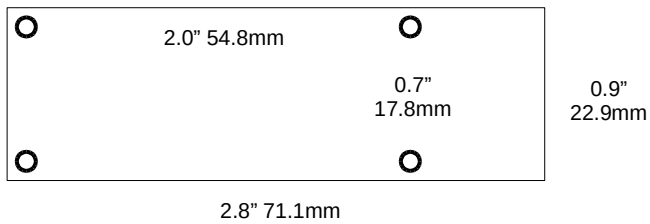
ALTS1-50K/ALTS2
