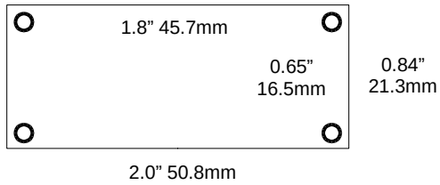
StratoLoggerCF
