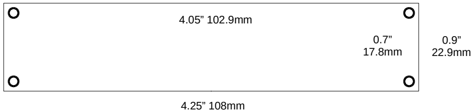
ALTS1-50K/ALTS2
